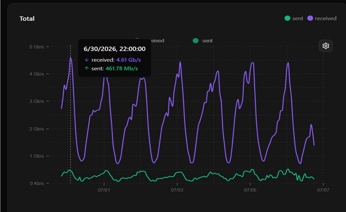
Figura 1. Monitoreo agregado de utilización de los enlaces principales.
